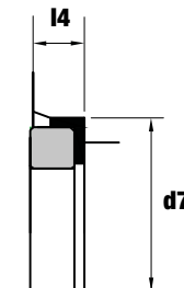
Dimensioni EN 12756 G60 QV (SILICIO/FKM)
