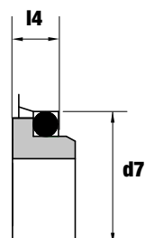
Dimensioni EN 12756 G6 QV (SILICIO/FKM)
