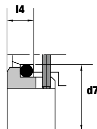
Dimensioni EN 12756 G9 BV (GRAFITE/FKM)
