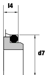
Dimensions EN 12756 G6 QV (SILICON/FKM)
