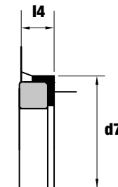
Dimensions EN 12756 G60 QV (SILICON/FKM)
