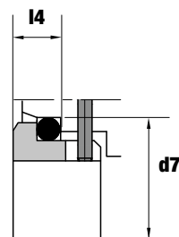
Dimensions EN 12756 G9 BV (GRAPHITE/FKM)
